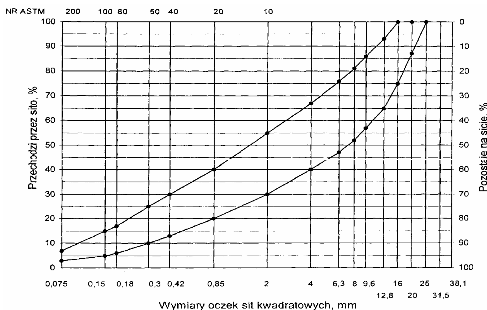
Rys. 2. Krzywe graniczne uziarnienia mieszanki mineralnej BA od 0 do 20 mm do warstwy wyrównawczej
