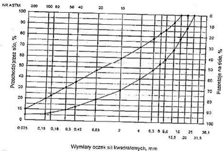
Rys. 1. Krzywe graniczne uziarnienia mieszanek mineralnej BA od 0 do 20 mm do warstwy ściernalnej nawierzchni drogi o obciążeniu ruchem dla KRI lub KR2
