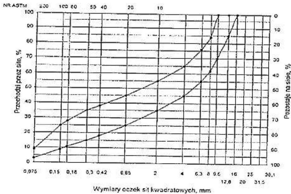
Rys. 10. Krzywe graniczne uziarnienia mieszanki mineralnej BA od 0 do 12,8 mm do warstwy wiążącej, wyrównawczej i wzmacniającej nawierzchni drogi o obciążeniu ruchem KRI lub KR2
