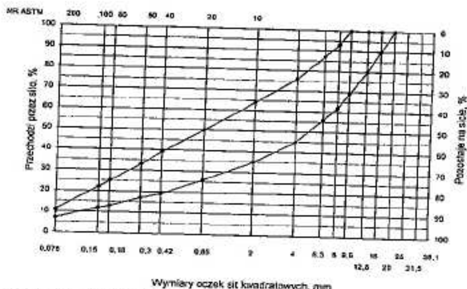
Rys. 2. Krzywe graniczne uziarnienia mieszanki mineralnej BA od 0 do 16mm, od 0 do 12,8 mm do warstwy ściernalnej nawierzchni drogi o obciążeniu ruchem KRI lub KR2
